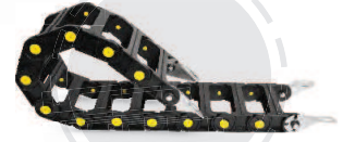
SAR-07010 120x50 Hortum Taşıyıcı
